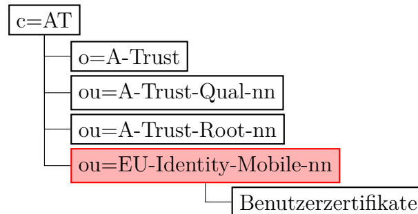
Abbildung 2: A-Trust Verzeichnisbaum
